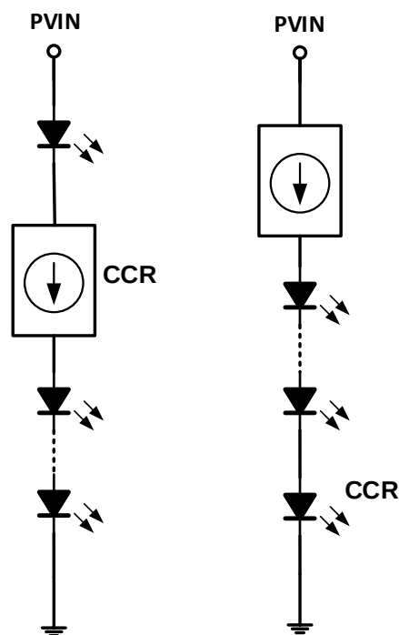
图 1. 典型应用电路
