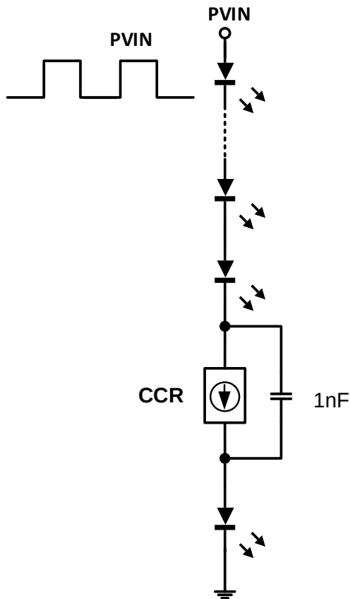
图 4. 调光应用
