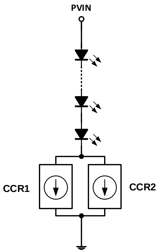
图 3. 多芯片并联使用
